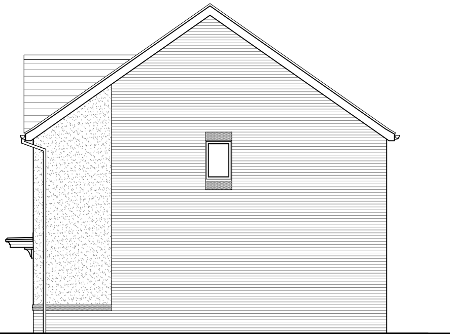
OXF.TF.2 (AS) SIDE ELEVATION
