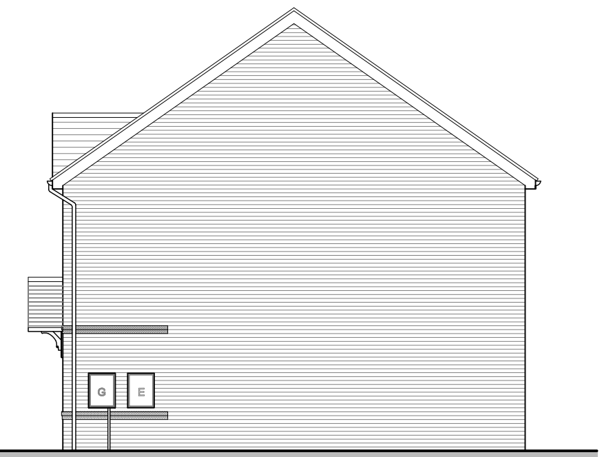
HIG.E.TF.1 (OPP) SIDE ELEVATION
