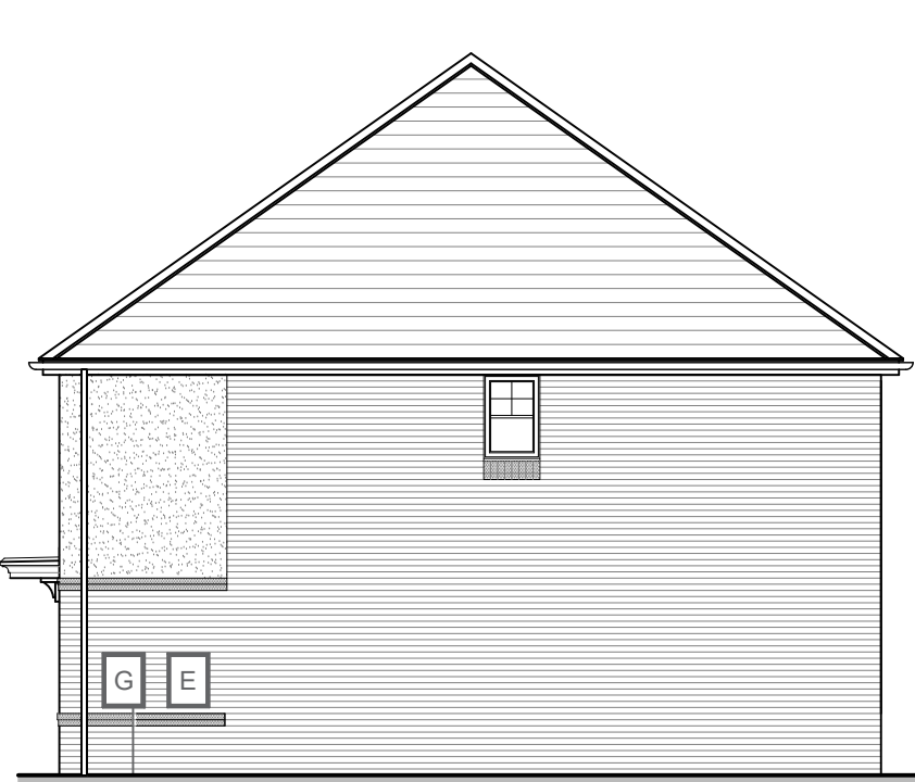
5P3B END (OPP) SIDE ELEVATION
