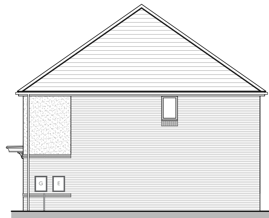
6P4B END (OPP) SIDE ELEVATION
