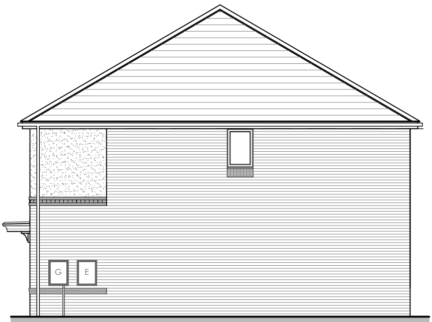
5P3B (OPP) SIDE ELEVATION
