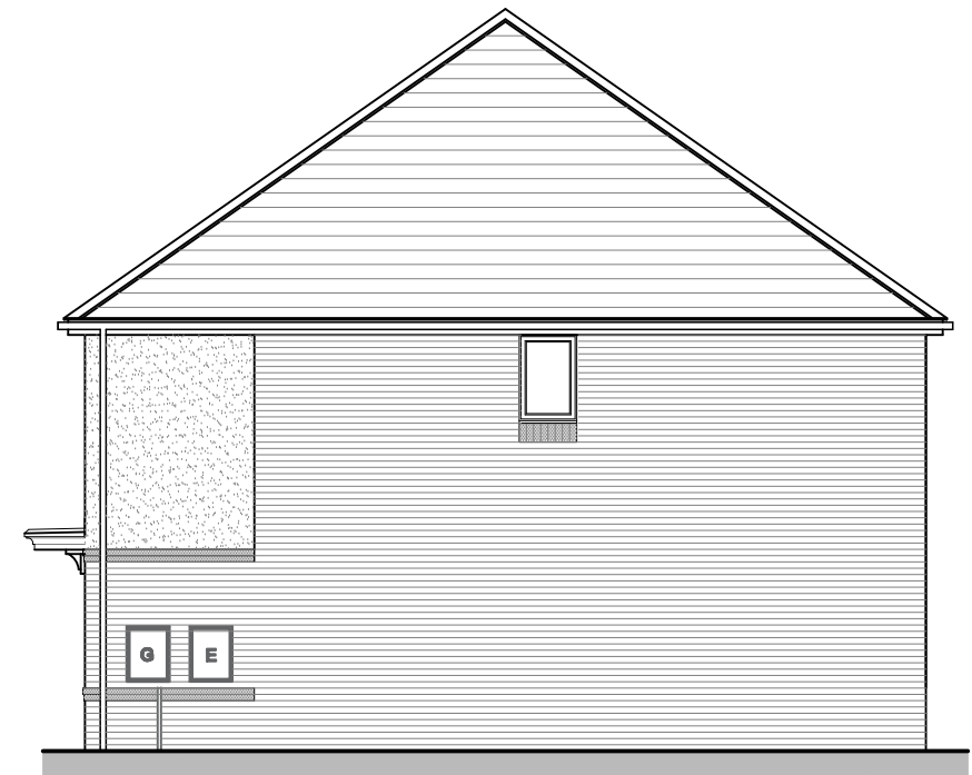
5P3B END (OPP) SIDE ELEVATION
