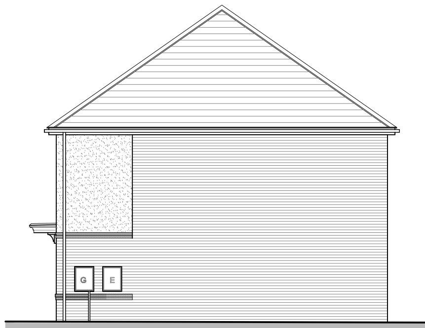
WARWICK (OPP) SIDE ELEVATION
