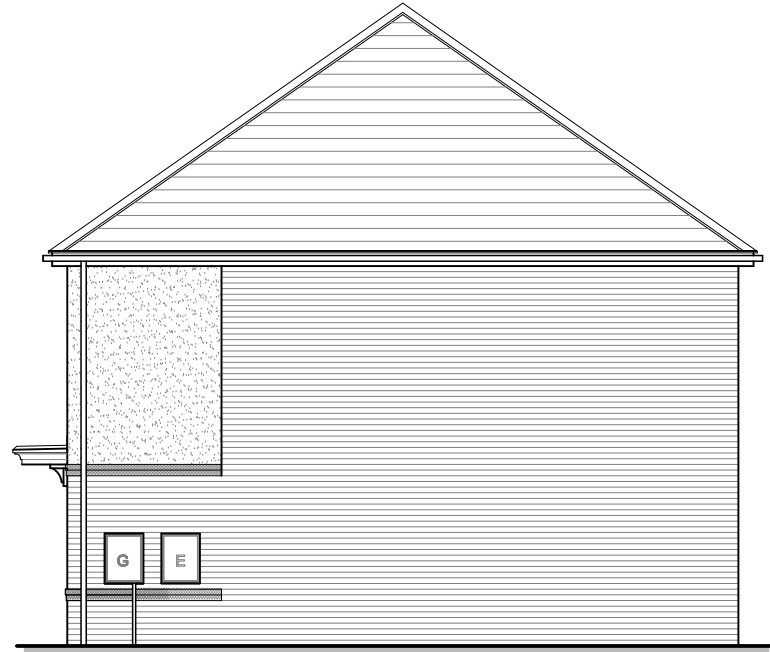
WARWICK (OPP) SIDE ELEVATION
