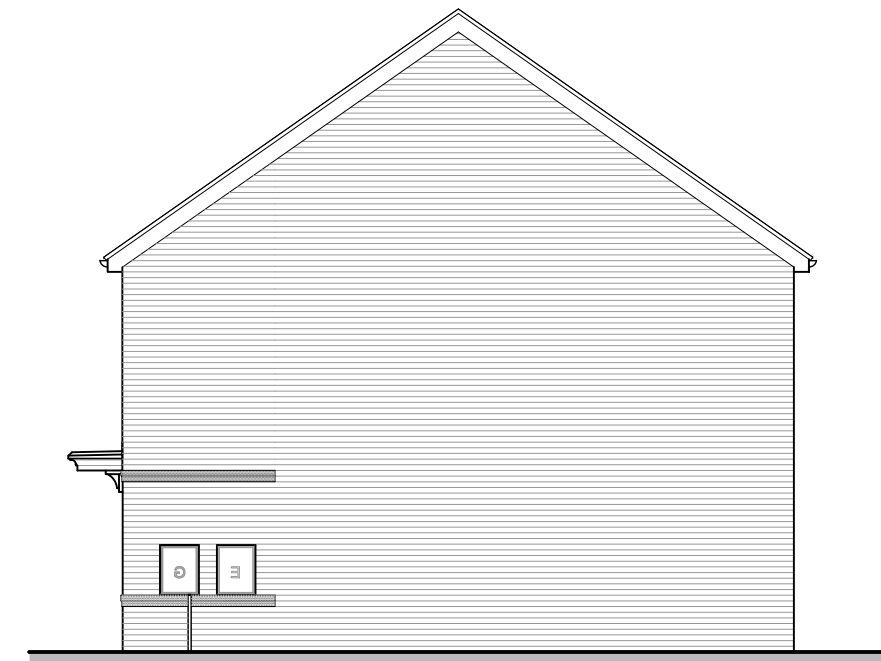
CLWYD END OPP SIDE ELEVATION
